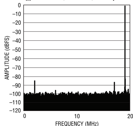
LTC2264-12: 8k Point FFT, f_{IN} = 139\text{MHz} , -1\text{dBFS} , 40\text{Mps}
